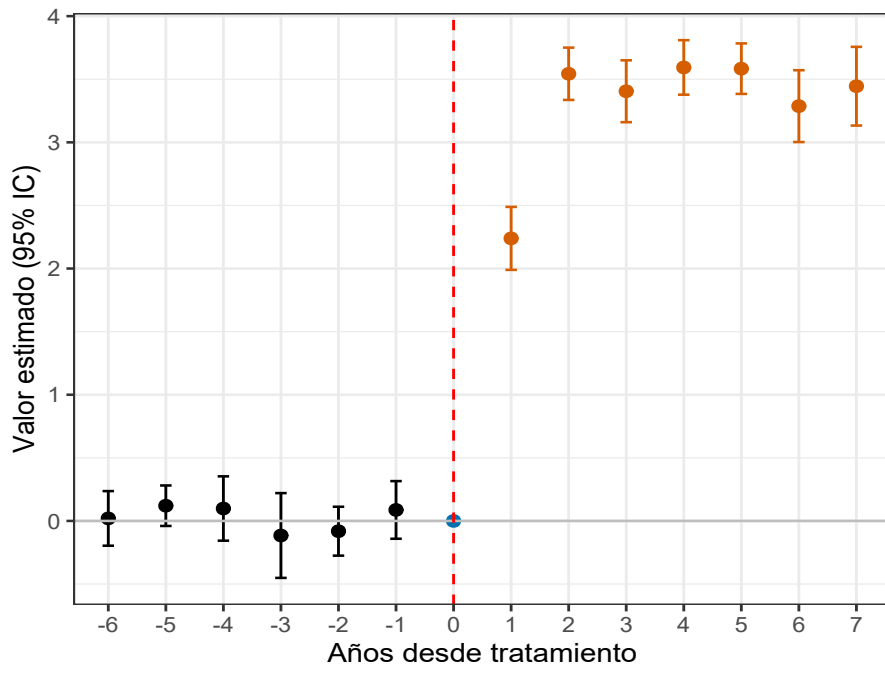
Figura 4: Gráfica DID
