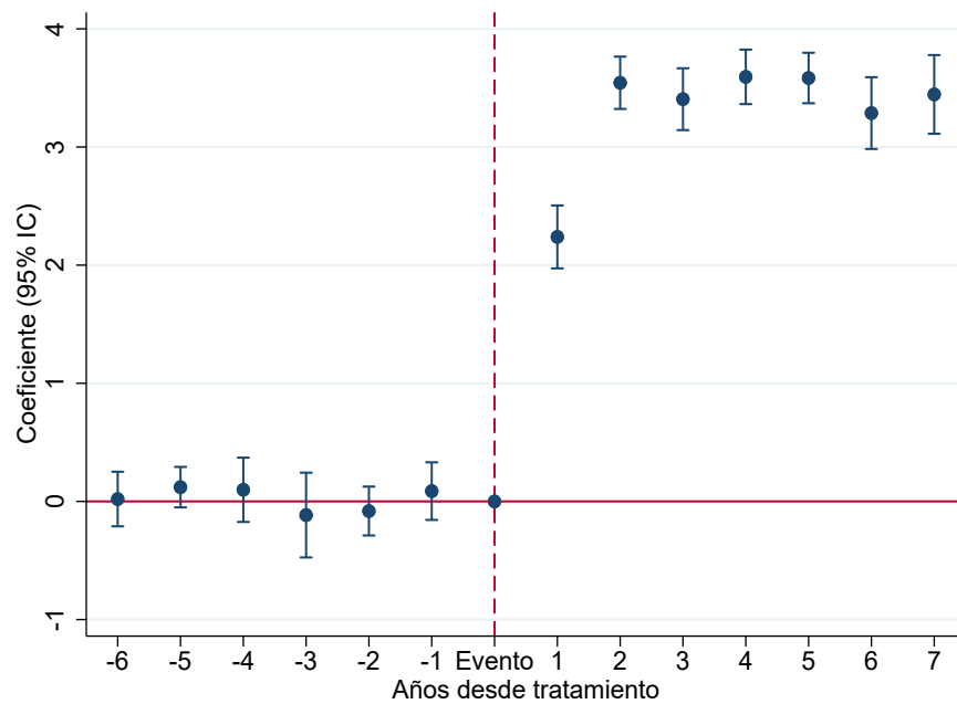
Figura 2: Gráfica DID
